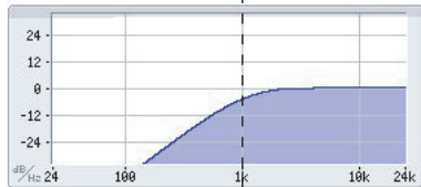
Hochpass (HPF)
